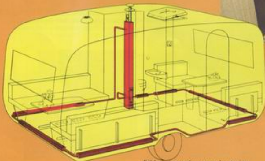
Bilde av sentralvarme anlegget i en Adria med konvektorer rundt vognen. Kondensfri oppvarming i hele vognen.
